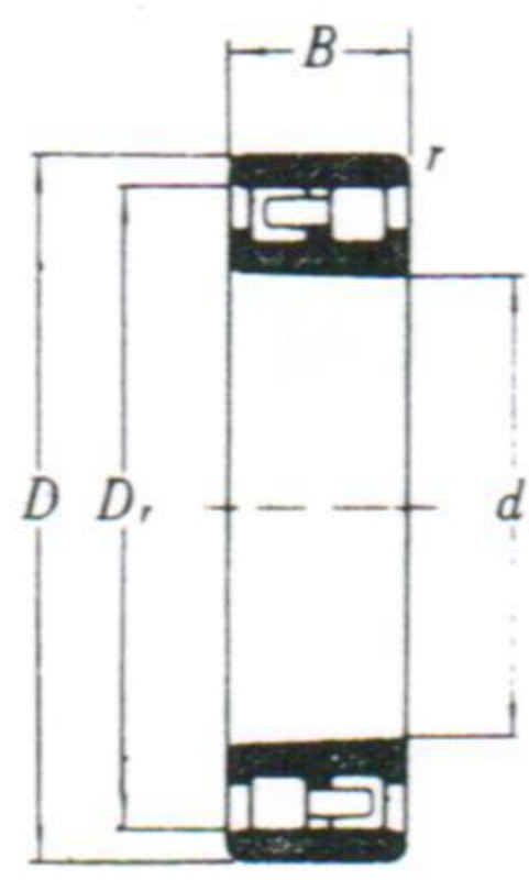
NN形 錐形內孔
