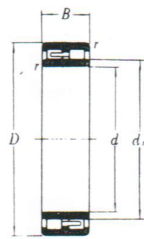
NNU形 圓筒內孔
