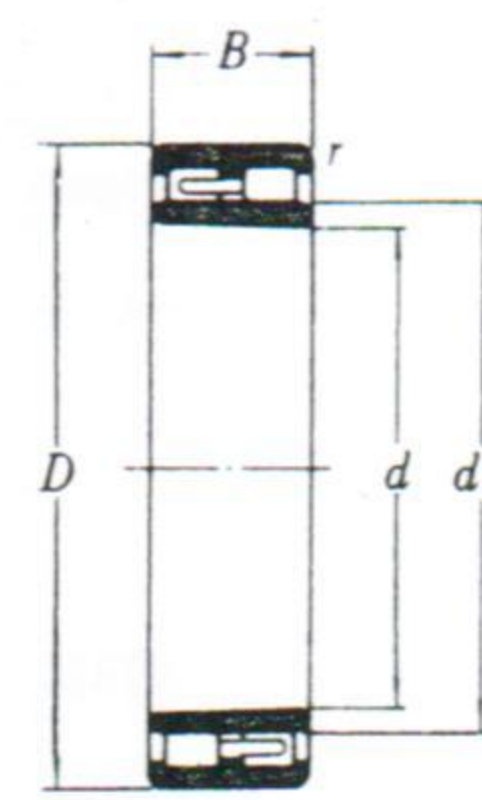
NNU形 錐形內孔
