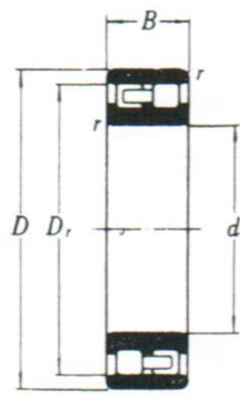
NN形 圓筒內孔
