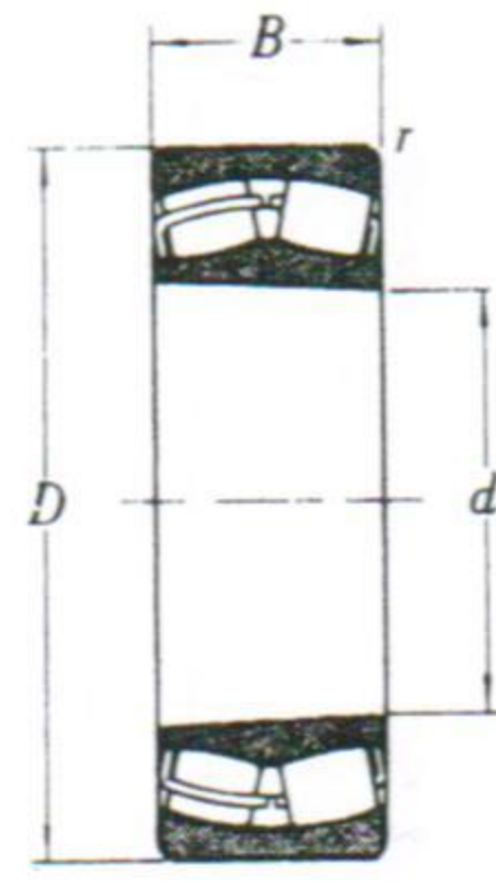
錐形内孔
